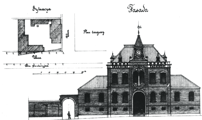
Projekt konkursowy na budowę strażnicy dla k. Miasta Podgórze (fragment) autorstwa Władysława Rausza – plan sytuacyjny i elewacja frontowa; w zbiorach ANK.
